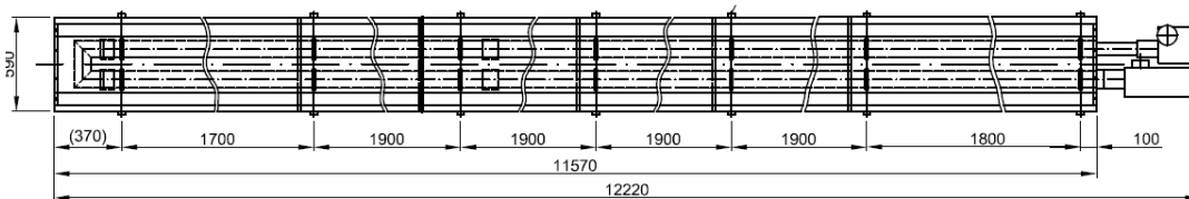
KM 45-U-12m
