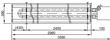
KM 10-U-3m
